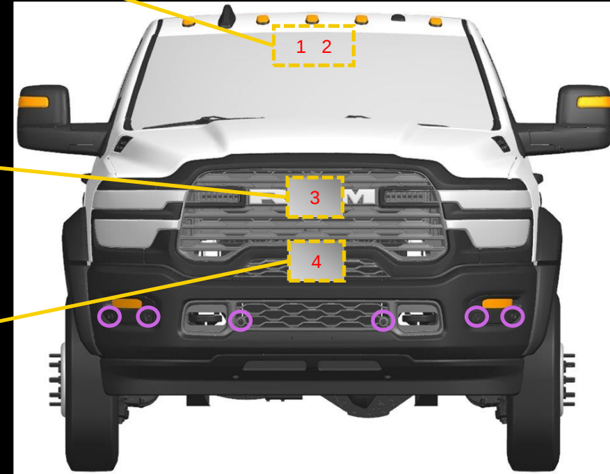
1 - Rain Sense Module 2 - Long Range Camera
